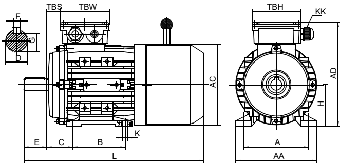
IM B3
