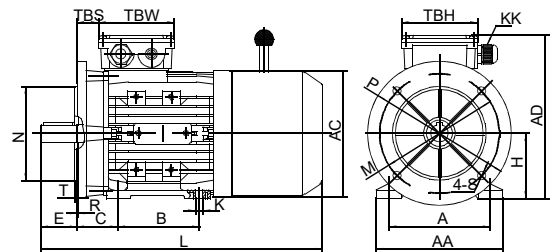
IM B35
