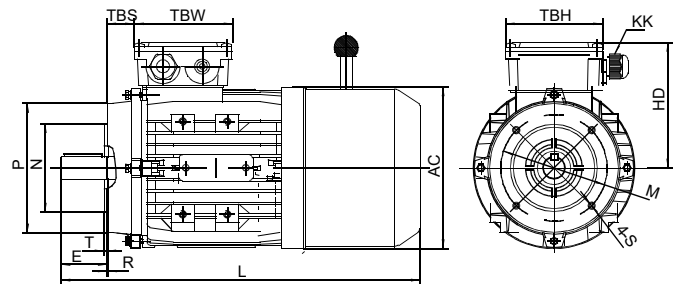
IM B14
