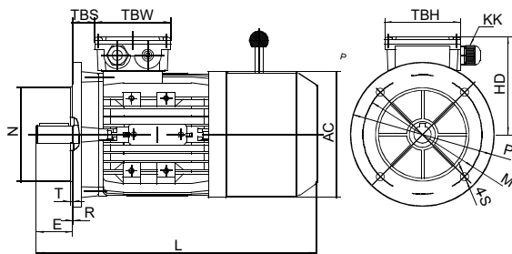
IM B5
