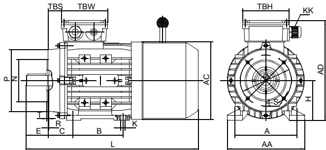
IM B34
